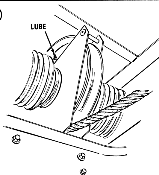
CABLE GUIDE
